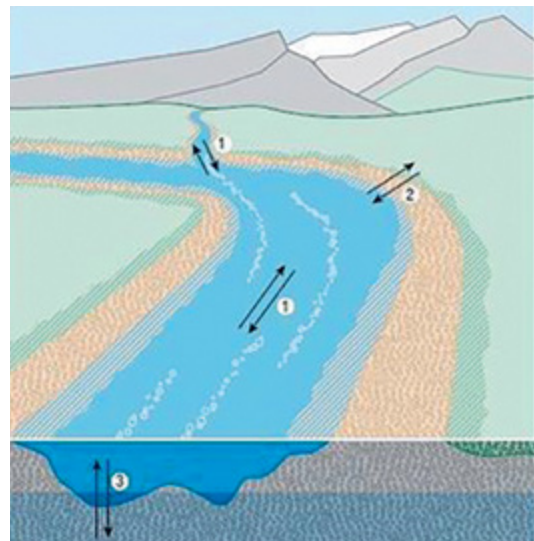
Schéma des connectivités d'une rivière.
